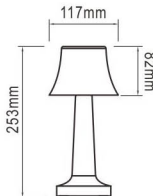
● ETLED-53D (Elmo)
